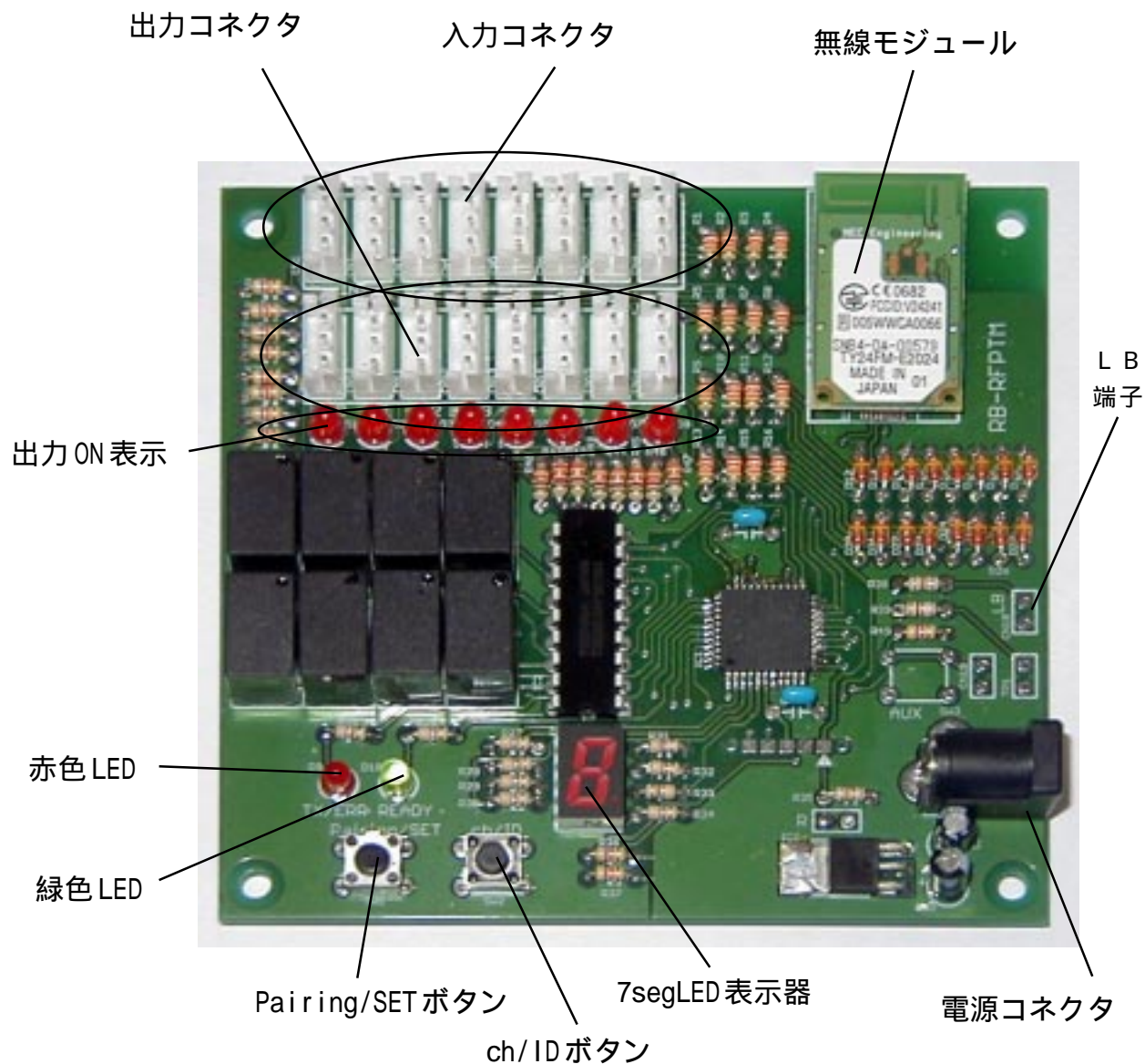
図5 : RB-RFPTM 基板
