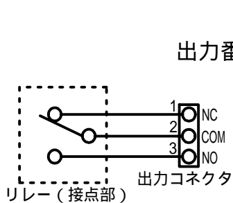
図7：出力等価回路
