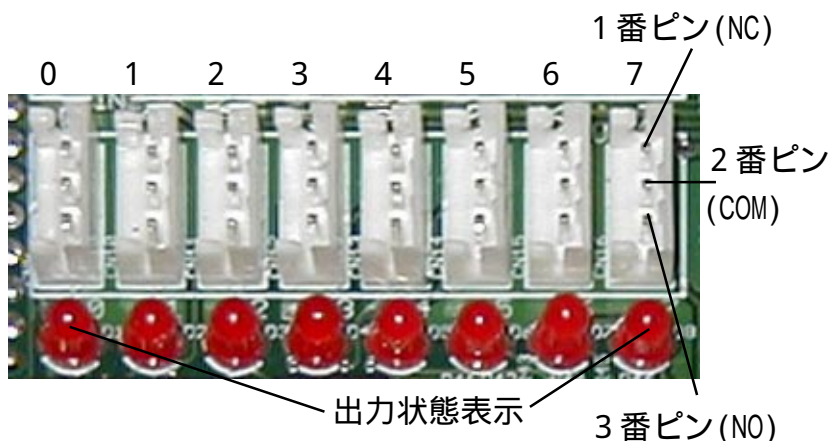
図8 親機出力コネクタの配置
