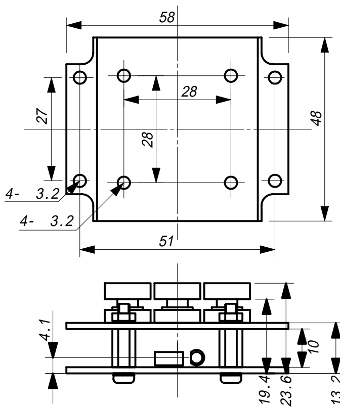
RB-RFRM 子機、ブロック寸法図
